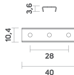
Sezione molletta di fissaggio
