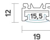
Sezione molletta di fissaggio
